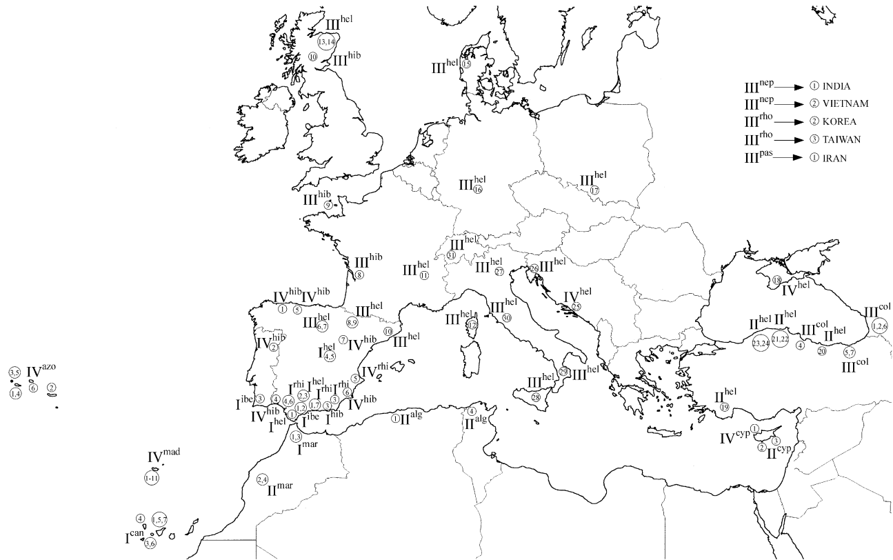
Fig. 5. Distributional map of the four Araliaceae chlorotypes (I, II, III, and IV) identified in Hedera (see text and Fig. 2). Species identification and circled population number as in Table 1. Abbreviations: alg, H. algeriensis ; azo, H. azorica ; can, H. canariensis ; col, H. colchica ; cyp, H. cypria ; hel, H. helix ssp. helix ; hib, H. hibernica ; ibe, H. maderensis ssp. iberica ; mad, H. maderensis ssp. maderensis ; mar, H. maroccana ; nep, H. nepalensis ; pas, H. pastuchovii ; rhi, H. helix ssp. rhizomatifera ; rho, H. rhombea .
